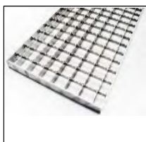
Podest dachowy - kratownica* , oczko: 30×30 mm, wysokość 25 mm, grubość 2 mm, zgodne z EN-516-1, nie zawiera mocowań
